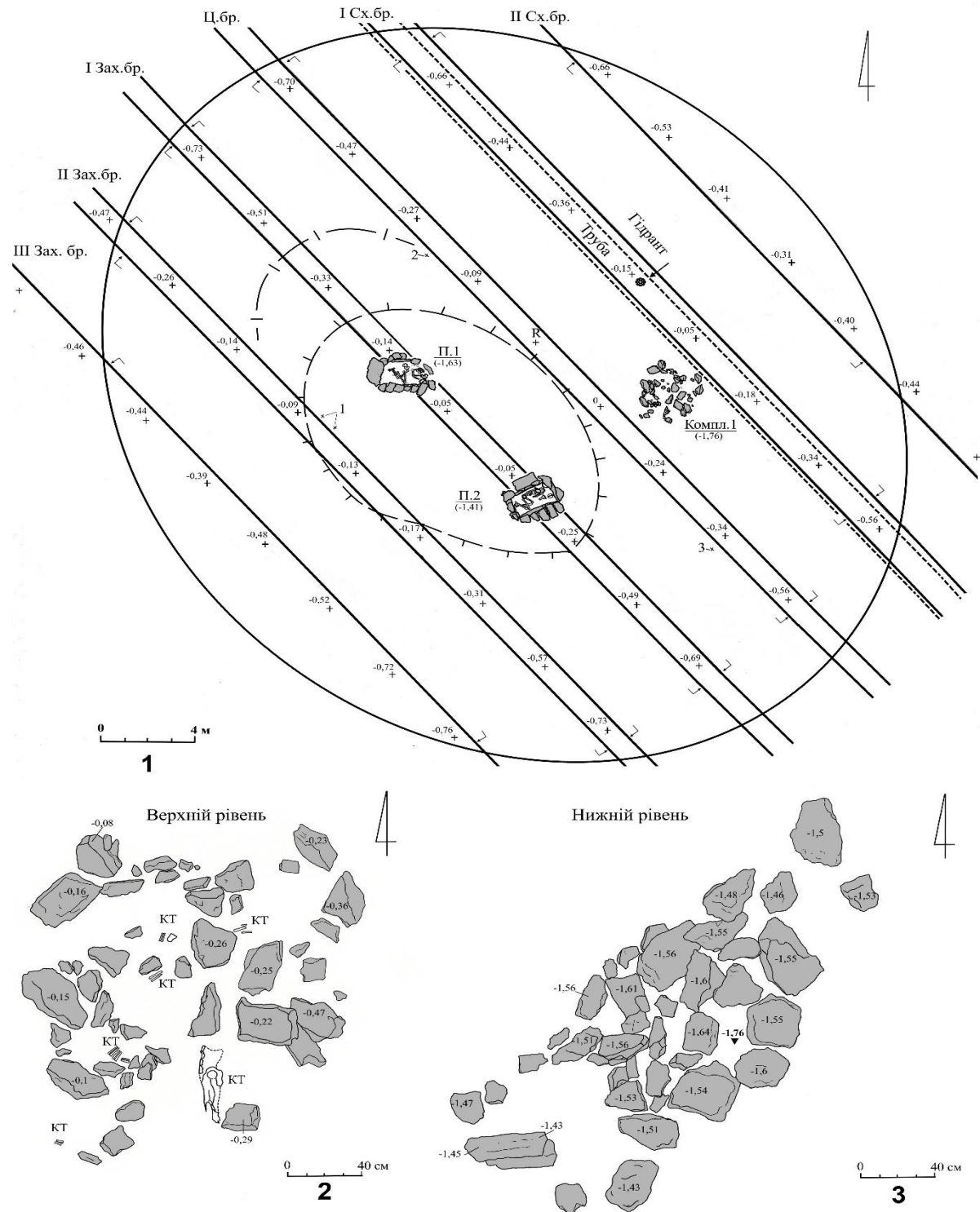
Рис. 6. Комишувате, курган 4. Загальний план кургану та комплекс 1 в насипу Fig. 6. Komyshevate, barrow 4. General plan of the barrow and complex 1 in the mound
