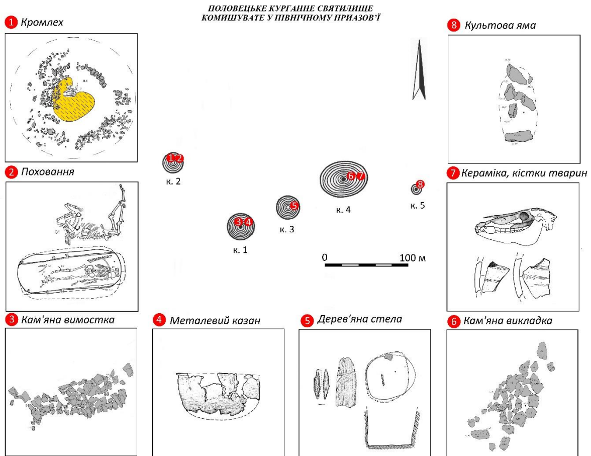
Рис. 10. Схема розташування артефактів кочівницького святилища середньовічного часу на курганному могильнику Комишувате
